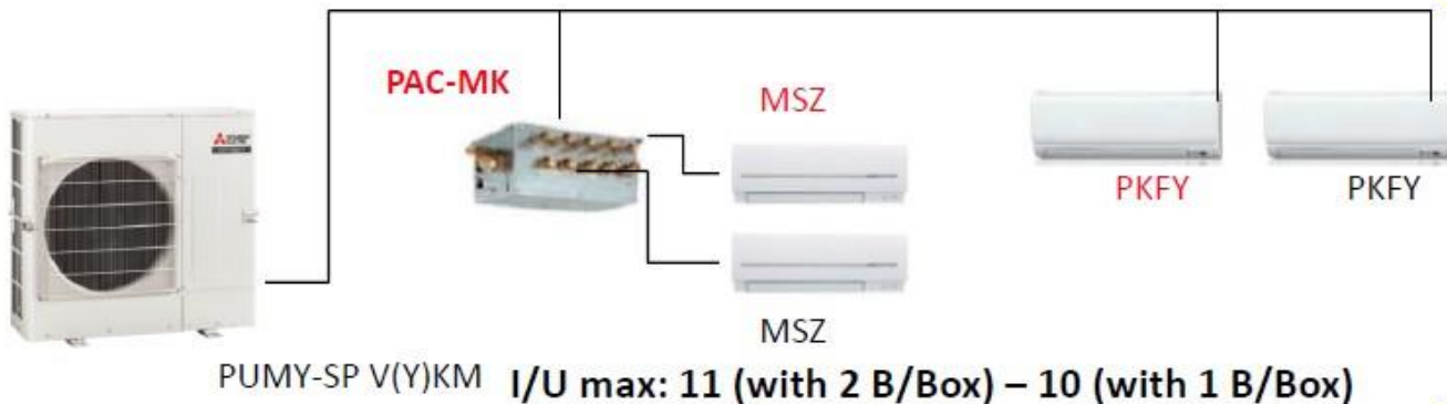
Skenari 3:Njesi VRF + Njesi multi me branch box
